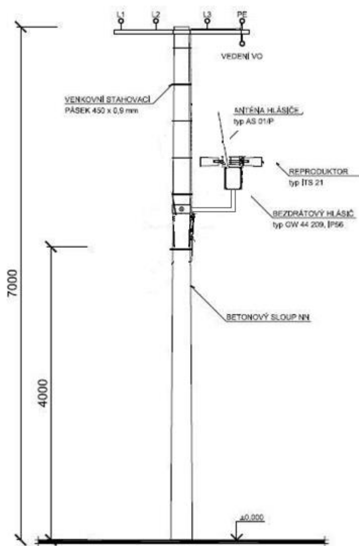
Obrázek 17: Schéma instalace bezdrátových hlásičů na výložníku betonového sloupu NN.
